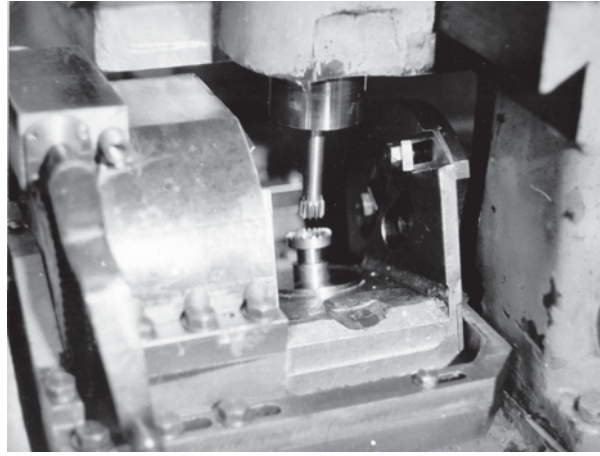
Fig. 11. Tallado del engranaje biparamétrico con el uso de una talladora de engranes.
