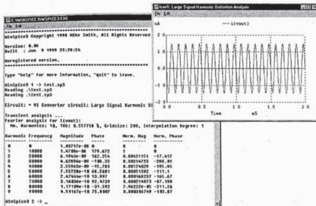
Figura 3: Simulación Pre/Post-Layout
