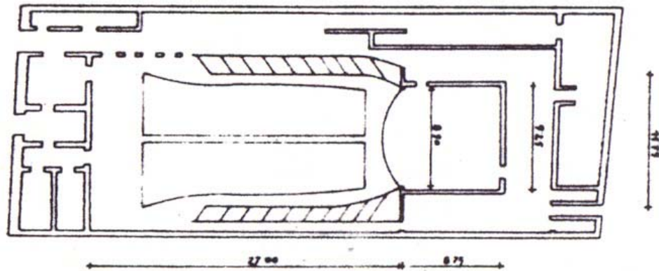
PLANTA DEL TEATRO CIRCO DE PAUL
